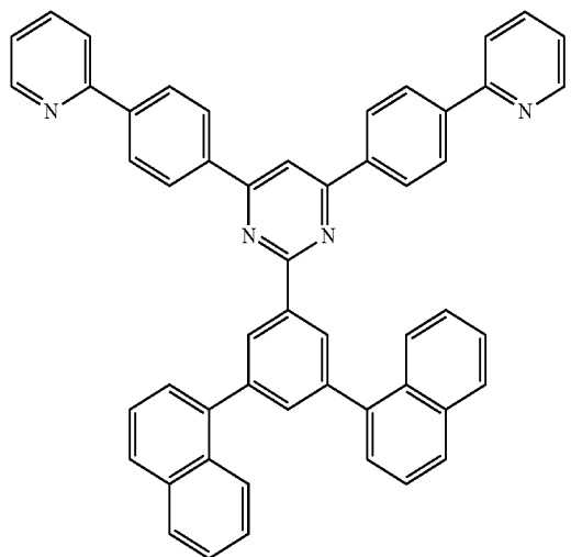
ET33
