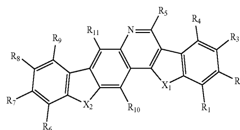
Formula 2E
