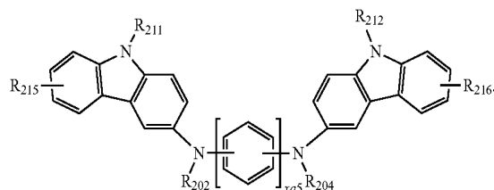
&lt;Formula 202A-1&gt;
