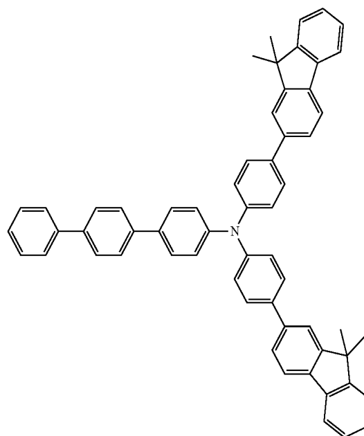
HT20
