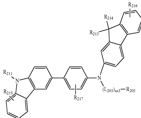
&lt;Formula 201A-1&gt;
