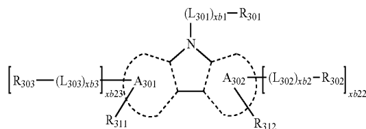
<Formula 301-1>
